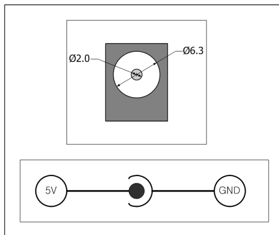
그림 1-7 DC 5V 전원 잭
