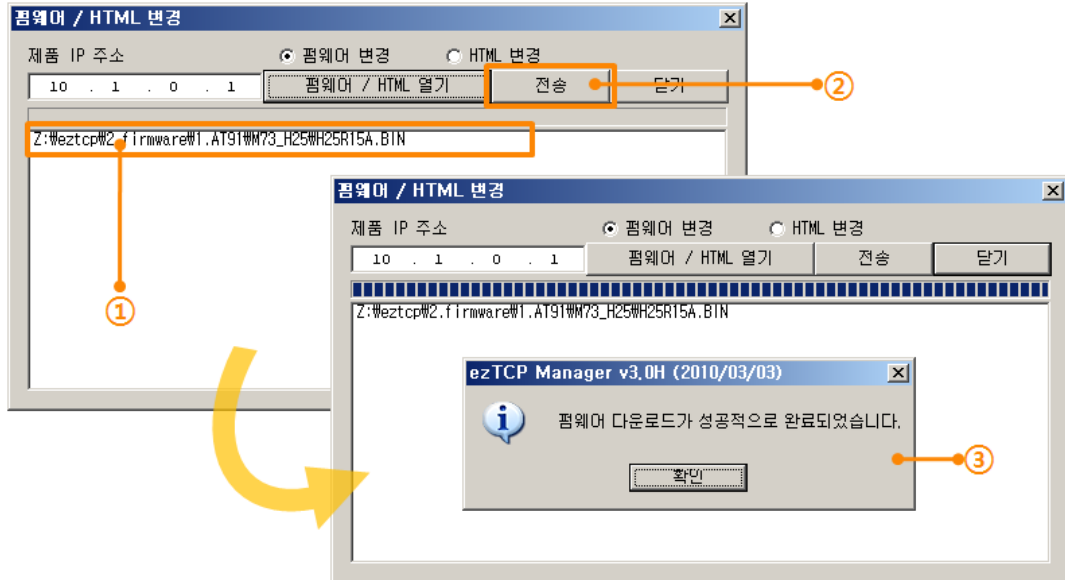
그림 6-2 펌웨어 전송
