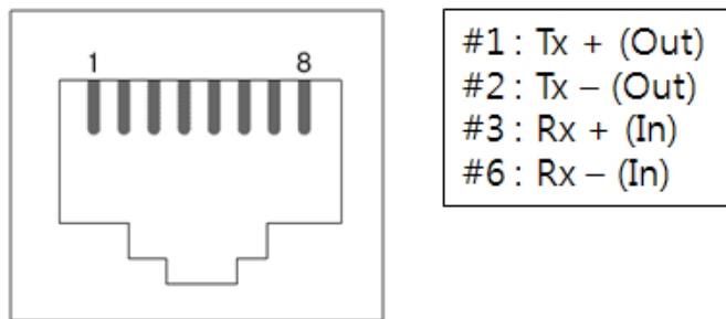
그림 1-6 RJ45 이더넷 커넥터 사양
