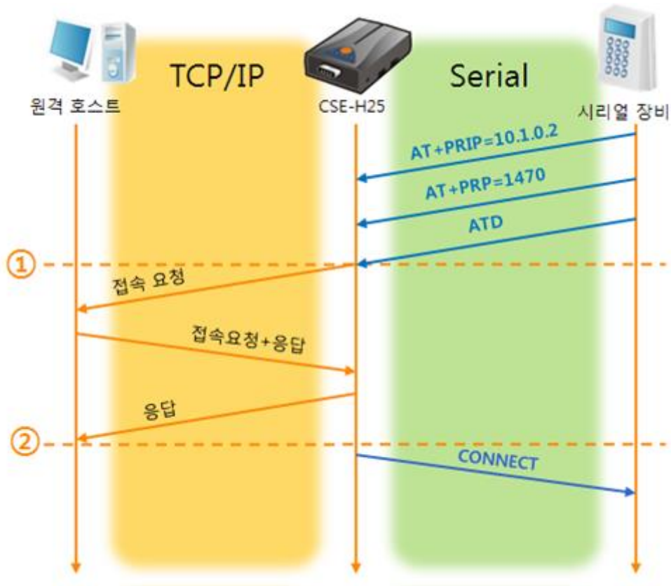
그림 5-8 TCP 능동접속
