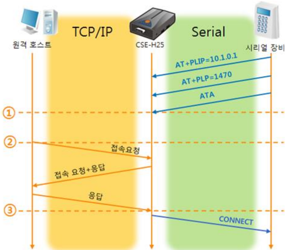
그림 5-7 TCP 수동접속
