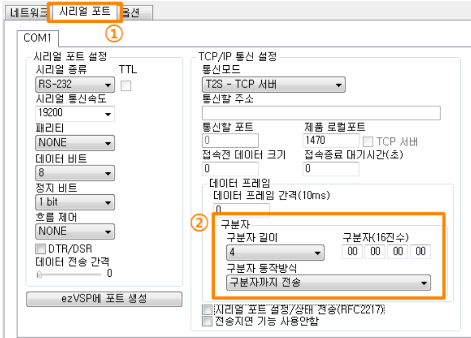
그림 7-4 구분자 설정
