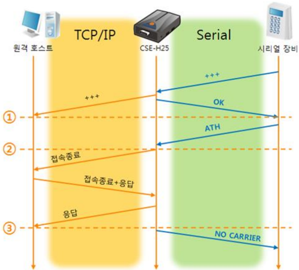
그림 5-9 TCP 접속종료
