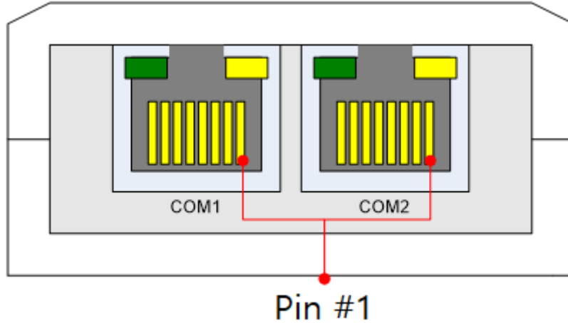
그림 2-1 시리얼포트용 RJ45 커넥터
