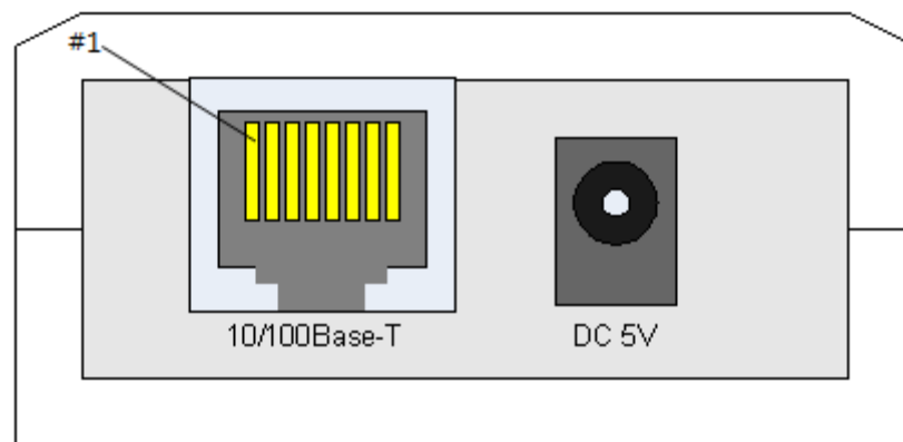
그림 2-2 이더넷 인터페이스
